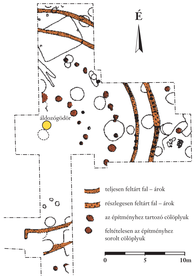
24. A körárok feltárt részének alaprajza. Füzesabony–Pusztaszikszó
