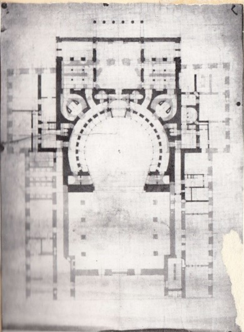
1. Átalakítási terv a pesti Német Színházhoz
