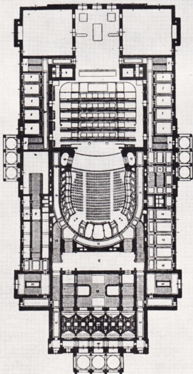
12. YBL MIKLÓS : AZ OPERAHÁZ ALAPRAJZA.
