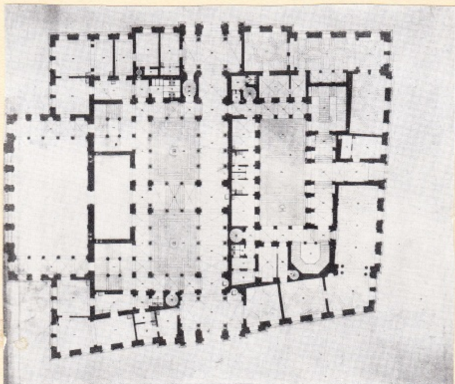
57. A Tudományos Akadémia pályaterve (alaprajz)
